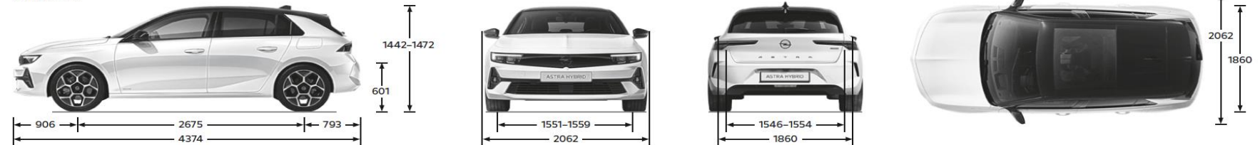
Astra 5-Türer Alle Maße in mm
