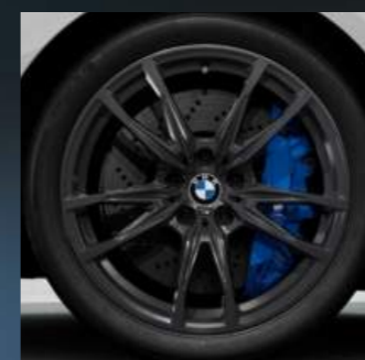
1T5 18"/19" M Schmiederäder Doppelspeiche 824 M, Orbitgrau
